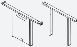
Middle Leg w/or w/o Cable Cover 中间脚带 / 不带走线盖 Single Bench 单边共享台 W:600,700 H: 720 Double Bench 双边共享台 W:1200,1400 H: 720
