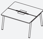
Double Bench 双边共享台 W:1200,1400,1500,1600,1800 D: 600,700 H: 750
