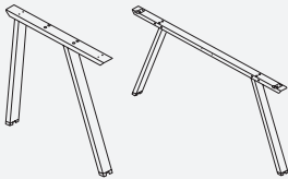
Trapezoid Leg 梯形台脚 Single Bench 单边共享台 W:600,700 H: 720 Double Bench 双边共享台 W:1200,1400 H: 720
