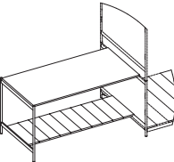
Social Table 社交高桌 W: 1630, 2030 D: 1090 H: 1050
