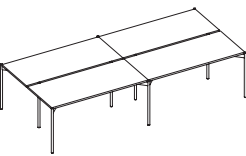
Bench 共享台 W: 1230, 1430, 1530, 1630 D: 1290, 1490, 1590 H: 740
