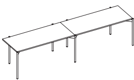
Single Bench 单边共享台 W: 1230, 1430, 1530, 1630 D: 660, 760, 810 H: 740
