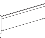
Acrylic Center Screen 亚克力正面屏风 W: 830, 1030, 1130, 1230 D: 30 H: 460
