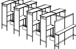
8 Clusters Touchdown 八人临时工作亭 W5170 D2100 H1920
