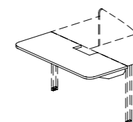
Extension Top, End 延伸台 W: 1200,1400,1600 D: 600
