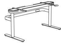
Fixed Leg for Single Desk 独立桌固定脚架 W: 1400,1500,1600,1800 D: 600,700
